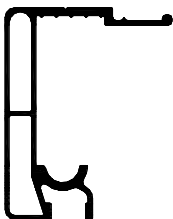
2548 Trilho Superior
