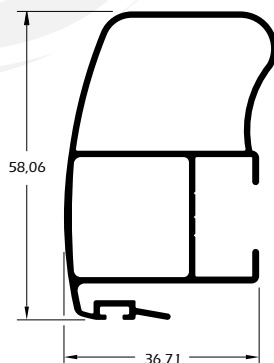
MG25-789 0,774 Kg/m Montante central com reforço sem baguete
