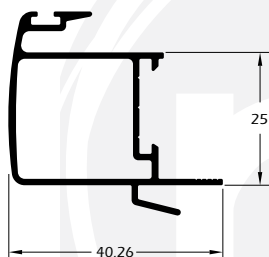
MG25-503 0,523 Kg/m Montante central intermediário da folha
