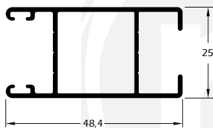
MG25-783 0,565 Kg/m Montante da folha sem baguete
