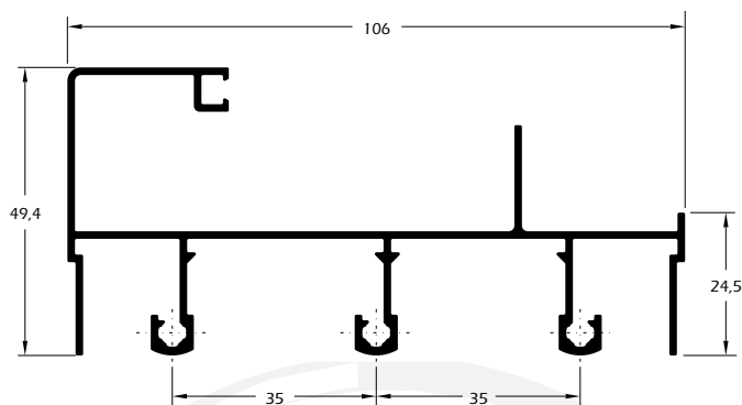
MG25-031 1,200 Kg/m Trilho superior correr 3 planos
