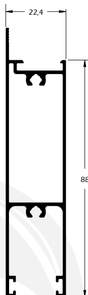
MG25-225 0,926 Kg/m Montante inferior da porta
