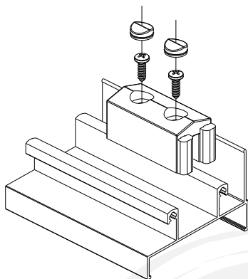
DETALHE DE APLICAÇÃO sem escala
