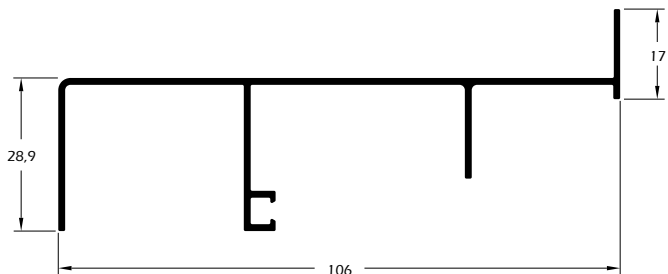
MG25-033 0,703 Kg/m Marco lateral correr 3 planos
