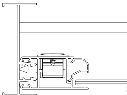
DETALHE DE APLICAÇÃO sem escala
