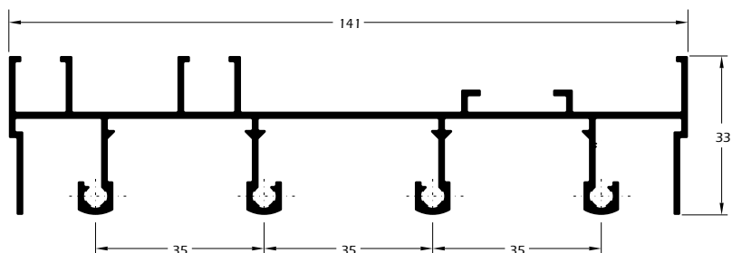
MG25-121 1,585 kg/m Trilho superior de correr 04 planos
