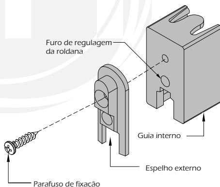
PERSPECTIVA sem escala
