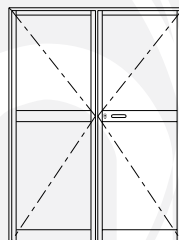
PORTA DE GIRO 2 FOLHAS
