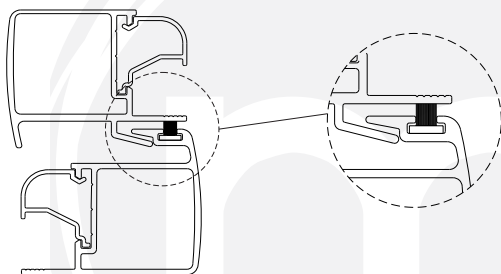
DETALHES DE APLICAÇÃO sem escala
