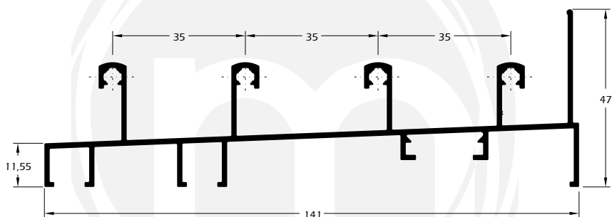
MG25-122 1,509 Kg/m Trilho inferior de correr 04 planos
