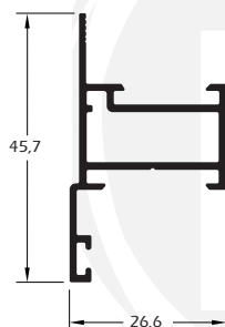
MG25-200 0,440 Kg/m Montante com escova maxim-ar
