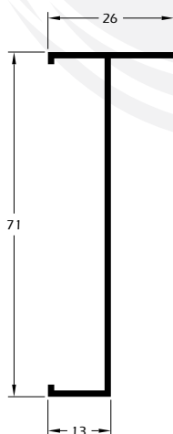
MG25-007 0,386 Kg/m Marco lateral liso de correr 2 planos
