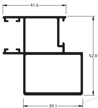
MG25-044 0,997 Kg/m Montante lateral / central da folha
