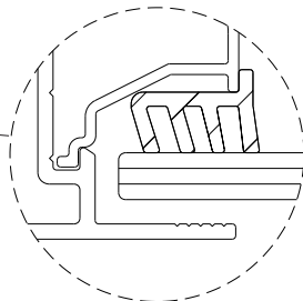
DETALHE DE APLICAÇÃO sem escala
