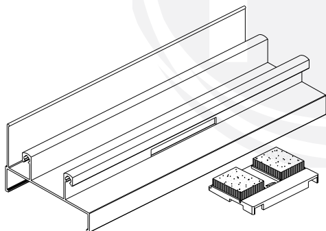
DETALHE DE APLICAÇÃO sem escala
