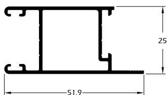
MG25-500 0,542 Kg/m Montante da folha com bagueete
