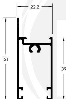
MG25-053 0,542 Kg/m Travessa da folha
