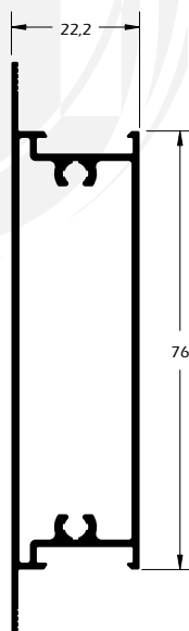
MG25-050 0,926 Kg/m Travessa intermediária da folha
