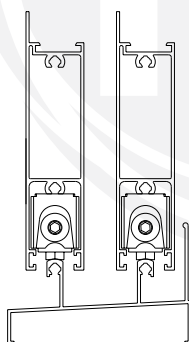
DETALHE DE APLICAÇÃO sem escala
