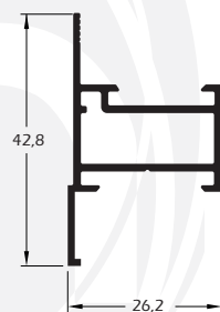
MG25-081 0,420 Kg/m Montante sem escova maxim-ar
