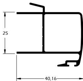
MG25-786 0,535 Kg/m Montante intermediário veneziana
