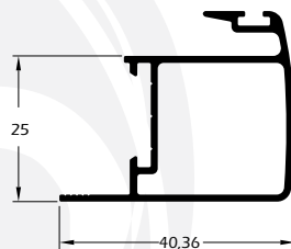
MG25-502 0,490 Kg/m Montante central externo da folha
