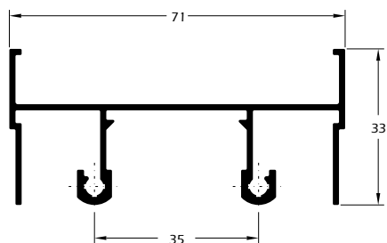
MG25-001 0,773 Kg/m Trilho superior de correr 02 planos
