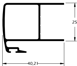
MG25-785 0,500 Kg/m Montante central veneziana
