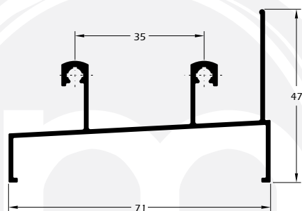
MG25-002 0,711 Kg/m Trilho inferior de correr 02 planos
