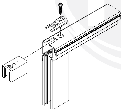
DETALHE DE APLICAÇÃO sem escala
