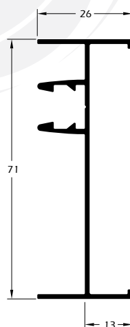
MG25-791 0,561 Kg/m Marco lateral correr 02 planos
