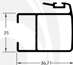
MG25-787 0,513 Kg/m Montante central sem baguete
