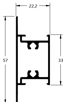
MG25-227 0,574 Kg/m Travessa intermediária da folha
