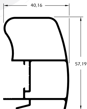
MG25-504 0,757 Kg/m Montante bi-tubular central interno
