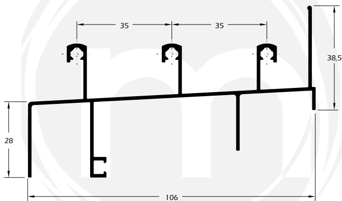
MG25-032 1,137 Kg/m Trilho inferior correr 3 planos
