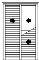
PORTA DE CORRER 3 FOLHAS COM VENEZIANA
