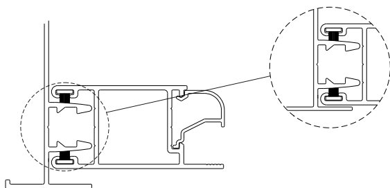
DETALHES DE APLICAÇÃO sem escala
