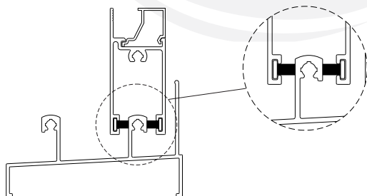
DETALHES DE APLICAÇÃO sem escala
