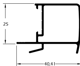
MG25-501 0,458 Kg/m Montante central interno da folha
