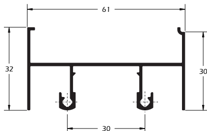
MG20-101 0,637 Kg/m Trilho superior de correr 02 planos
