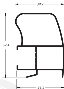
MG20-136 0,688 Kg/m Montante central interno com reforço
