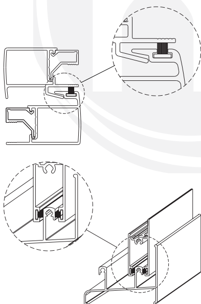
DETALHES DE APLICAÇÃO sem escala
