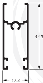
MG20-137 0,427 Kg/m Travessa folha correr sem baguete
