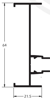
MG20-103 0,462 Kg/m Marco lateral correr 02 planos com contra fecho
