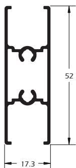
MG20-139 0,527 Kg/m Travessa intermediária folha sem baguete
